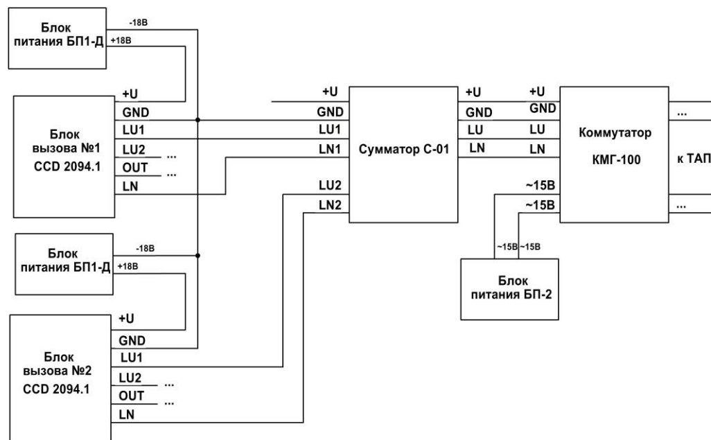
Рис. 2б Схема подключения сумматора с дополнительным источником питания, при величине сопротивления проводов, соединяющих блок вызова с сумматором более 6 Ом для ССД 2094.1 и более 1,5 Ом для ССД 2094.1/ПК (длинная линия)
